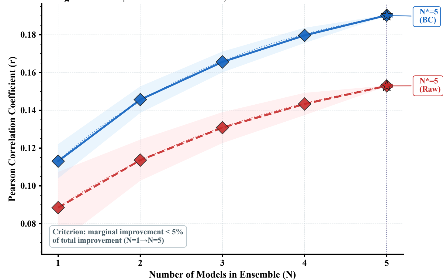
(d) Pearson Correlation Coefficient (r)
